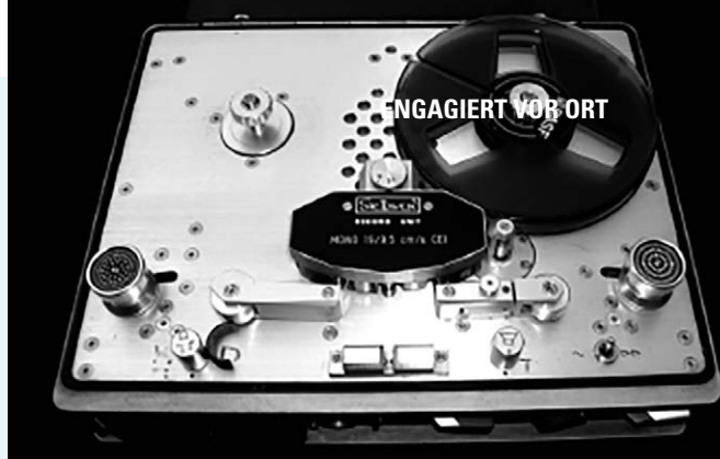
Aufnahmegerät „STELLAVOX“
